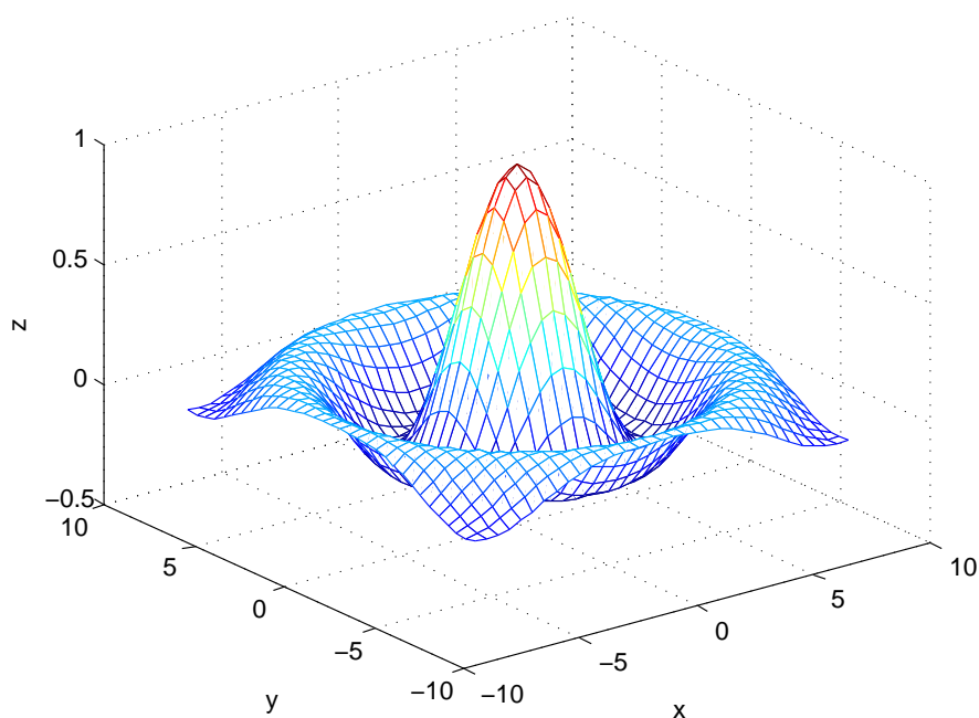
Rysunek 4.1. Przykładowy wykres trójwymiarowy.
